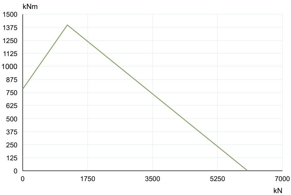
La Leonessa VE147A00 — Curva de capacidad de carga
