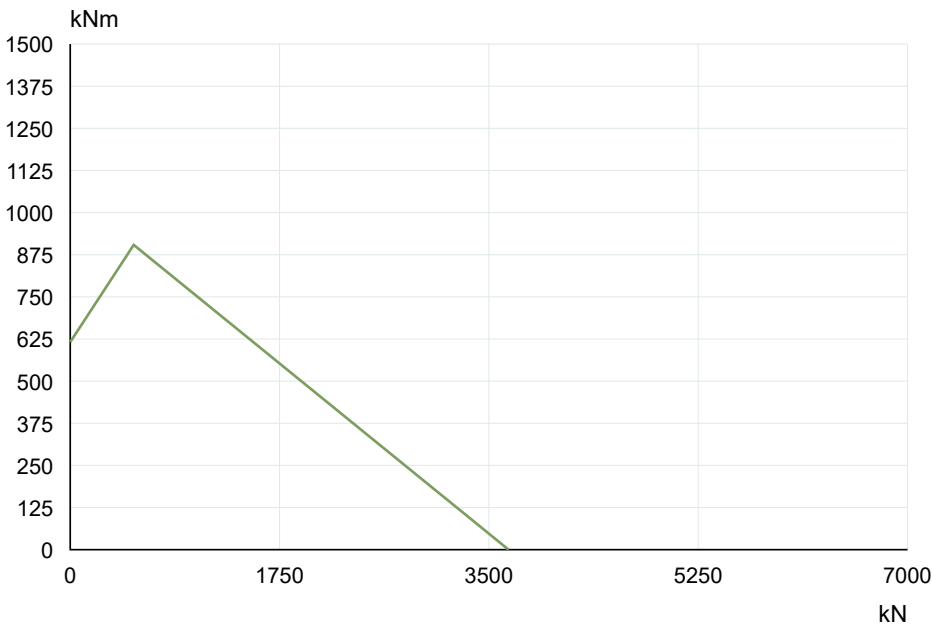
La Leonessa VE140A01 — Curva di capacità di carico
