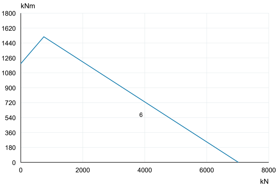
VE138B05 · Curva originale 2SE 6 · PDF p11
