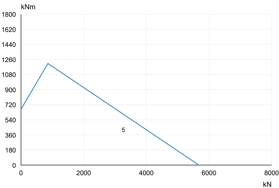
VE129B01 · Curva originale 2SE 5 · PDF p11
