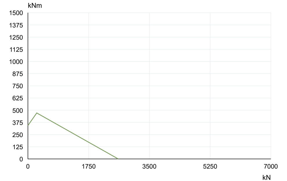
La Leonessa VE120A01 — Curva di capacità di carico
