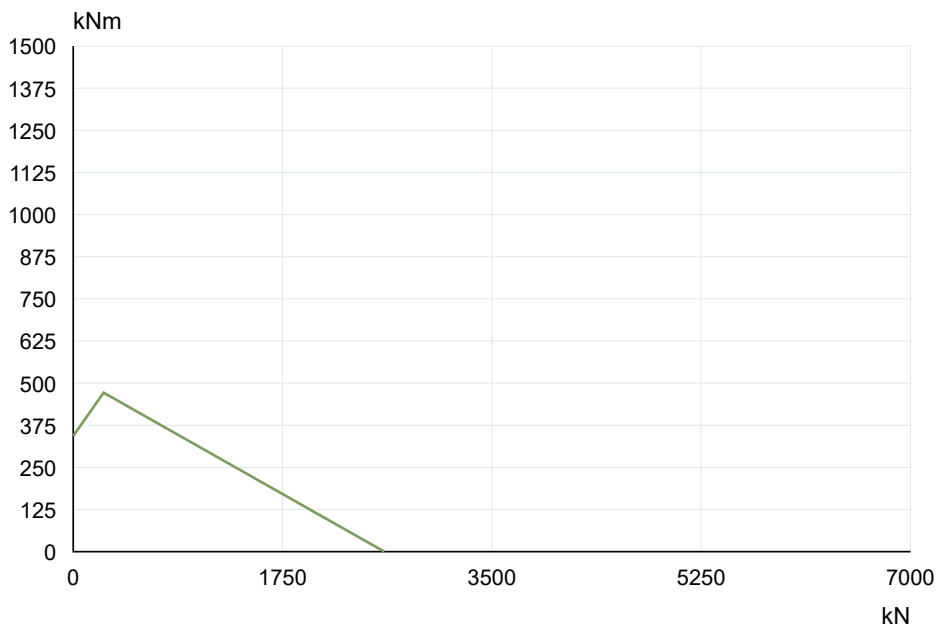
La Leonessa VE120A01 — Curva de capacidad de carga
