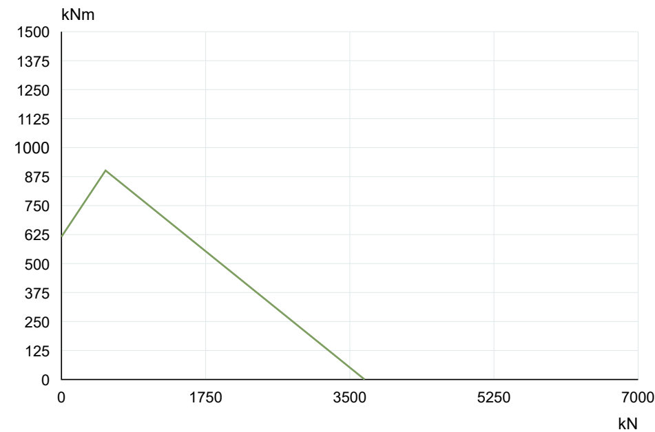
La Leonessa VE113A03 — Кривая несущей способности
