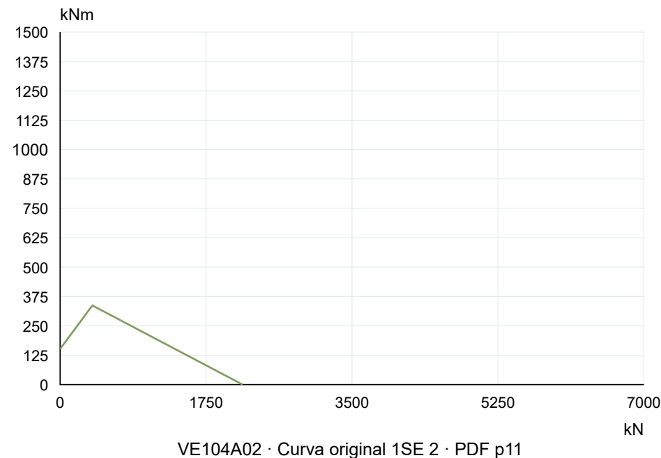
La Leonessa VE104A02 — Curva de capacidade de carga
