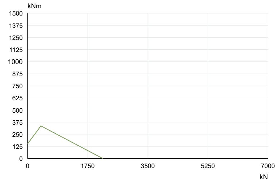
La Leonessa VE104A02 — Tragfähigkeitskurve
