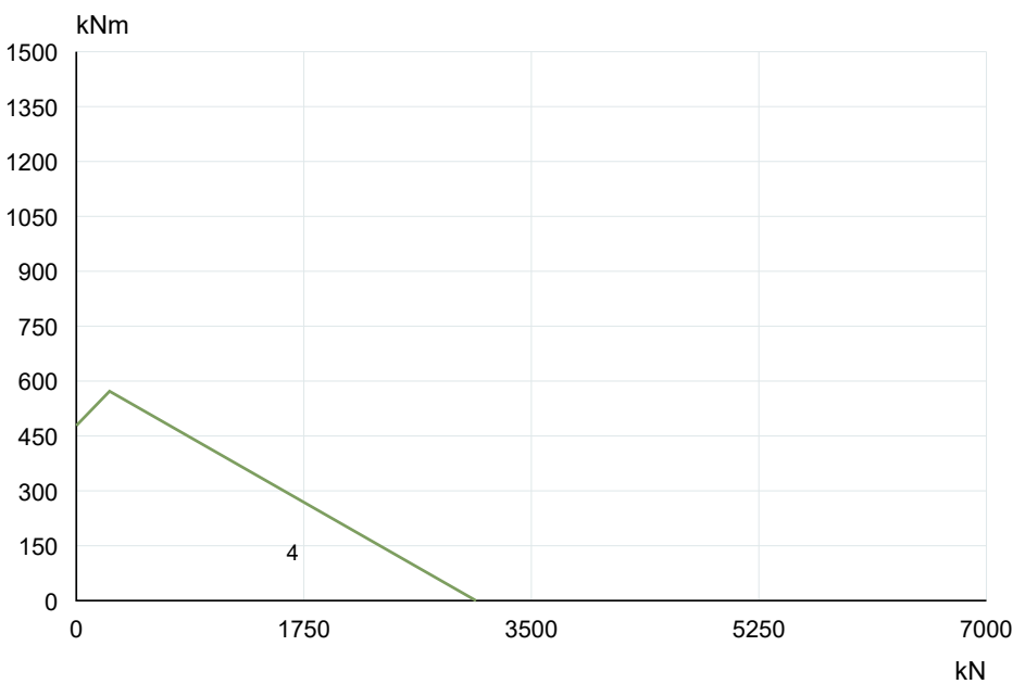
VE102A00 · Curva originale 1SE 4 · PDF p11
