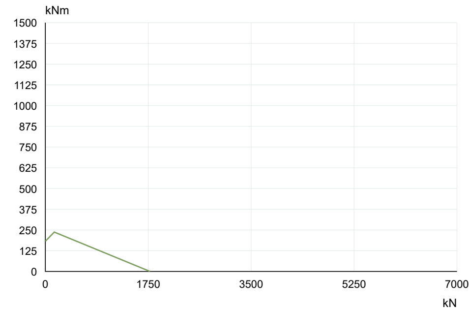
La Leonessa VE086A00 — Кривая несущей способности
