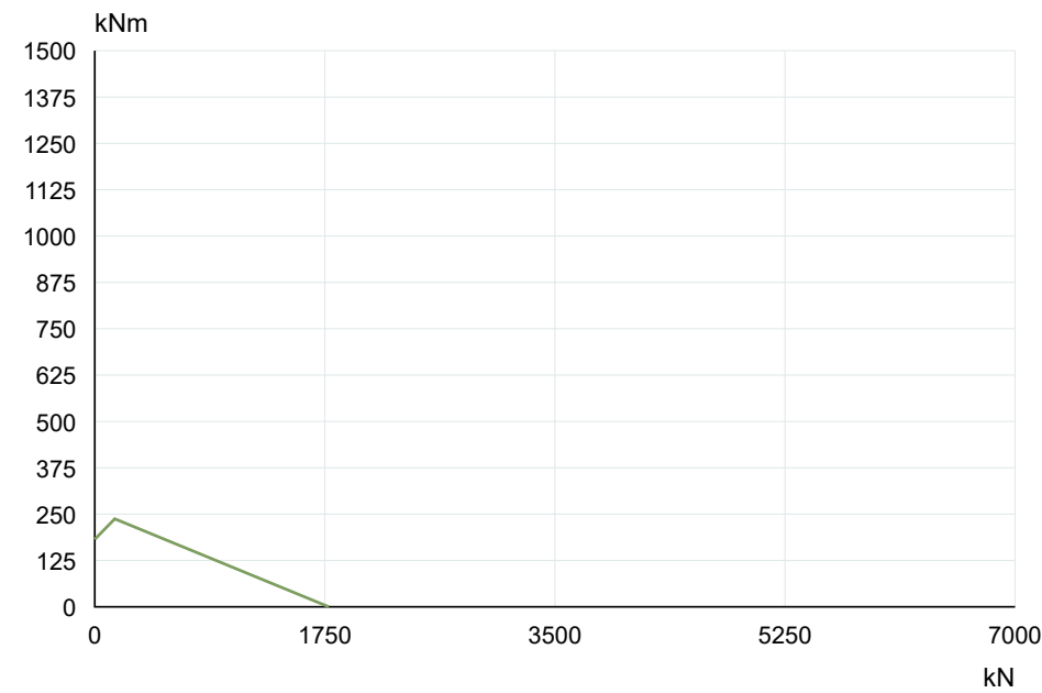
La Leonessa VE086A00 — Curva de capacidade de carga
