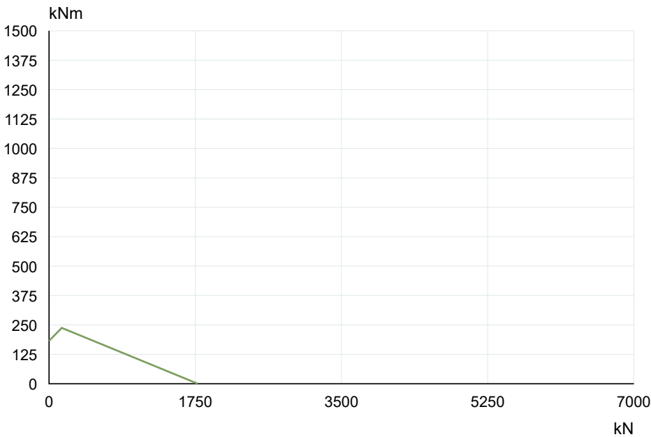
La Leonessa VE086A00 — Curva di capacità di carico
