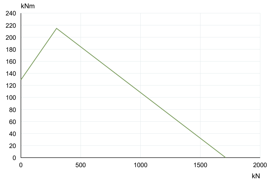
La Leonessa VE079A00 — Curva de capacidad de carga
