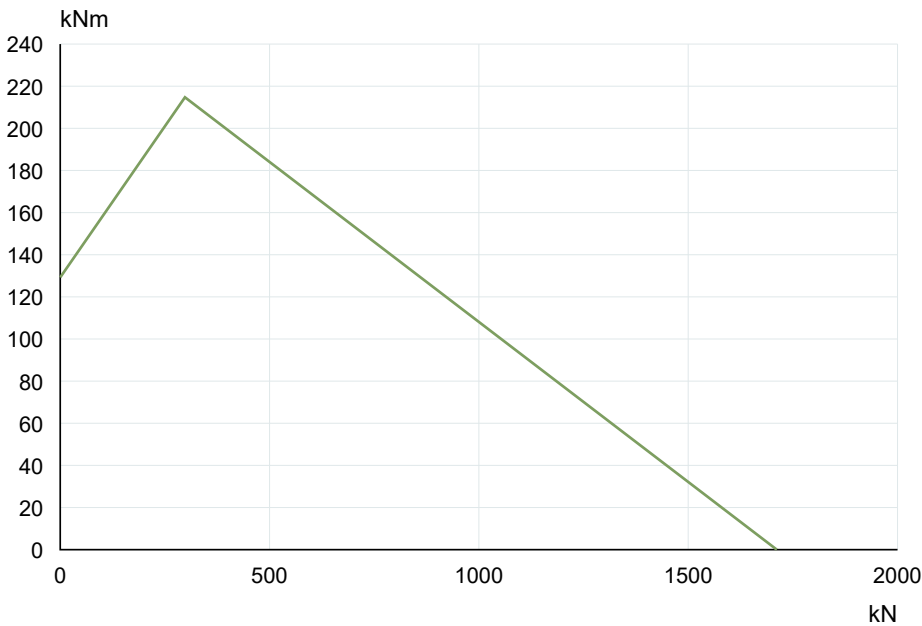
La Leonessa VE079A00 — Tragfähigkeitskurve
