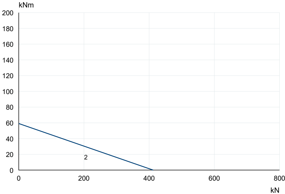
VE074Z100 · Curva originale Z 2 · PDF p4
