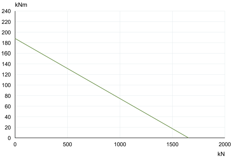
La Leonessa VE069A05 — Curva de capacidade de carga
