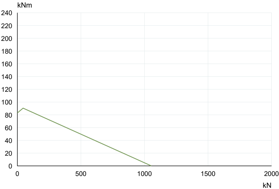
La Leonessa VE059A10 — Curva di capacità di carico
