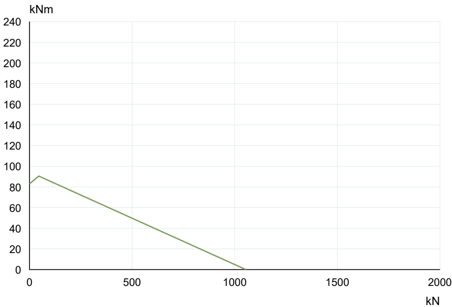
La Leonessa VE059A10 — Tragfähigkeitskurve
