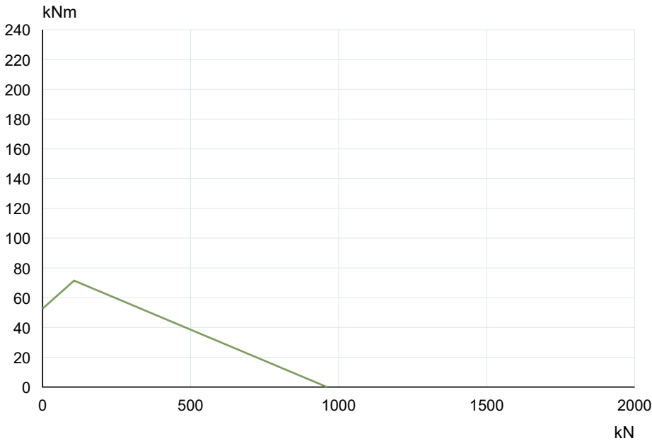
La Leonessa VE050A02 — Tragfähigkeitskurve
