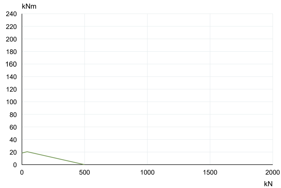
La Leonessa VE031A14 — Curva de capacidad de carga
