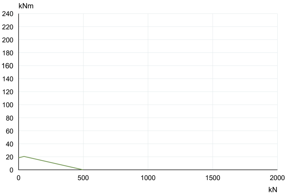
La Leonessa VE031A14 — Tragfähigkeitskurve
