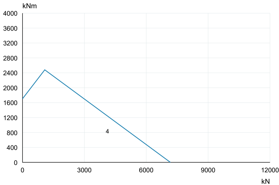
V40E027 · Curva originale 1RE 4 · PDF p15
