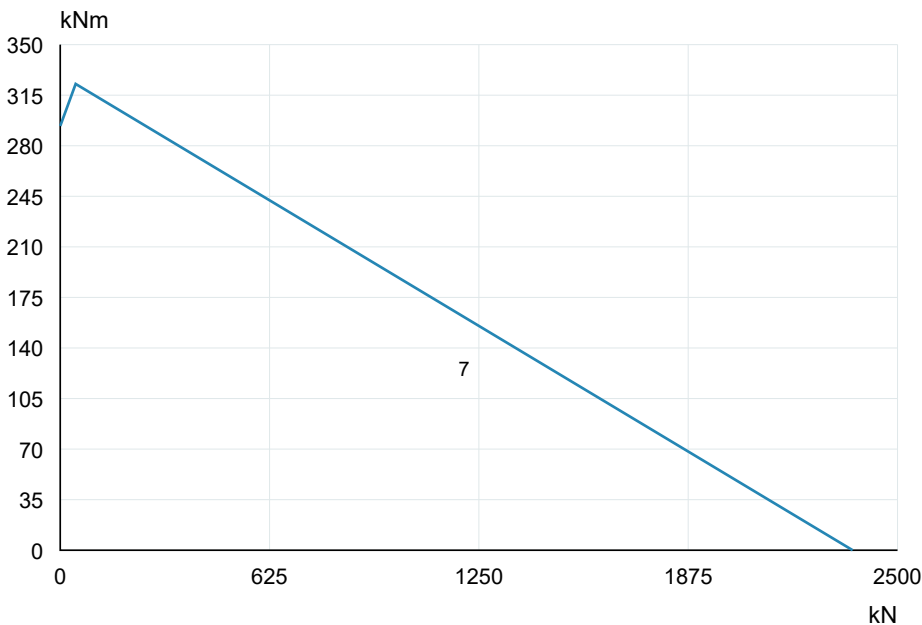
V30S026 · Curva originale 1R 7 · PDF p7
