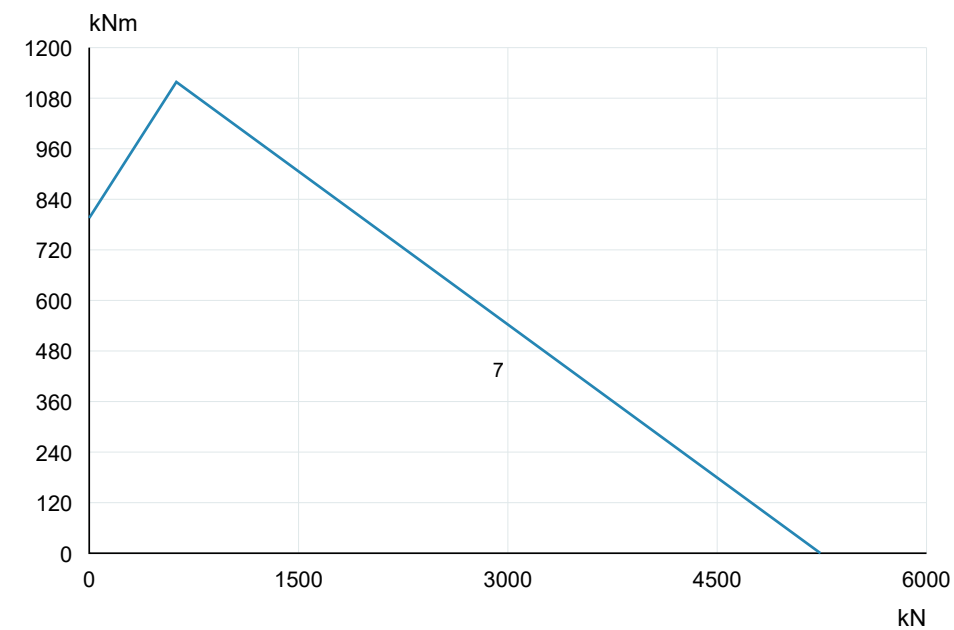
V30S023 · Curva original 1R 7 · PDF p11
