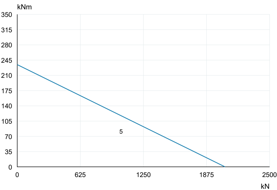
V25S090 · Curva originale 1R 5 · PDF p7
