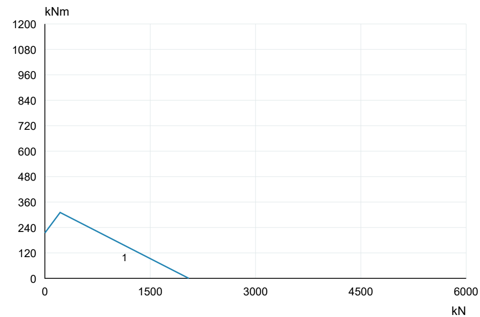
V25S085 · Curva original 1R 1 · PDF p11
