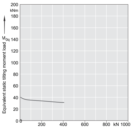
Крепёжные болты · Опорная нагрузка
